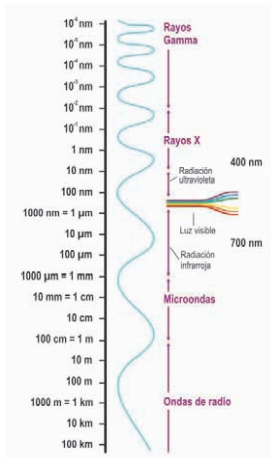
Figura 6. Espectro electromagnético.
